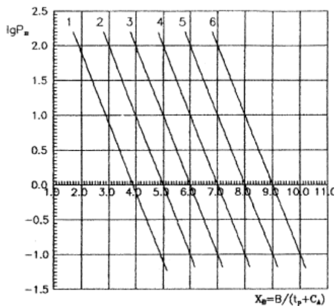
Рис. 8. Зависимость параметра \lg P_n для паров ЛВЖ от параметра x_6 = B/(t_p + C_A) при различных значениях параметра A : 1 - 3,9; 2 - 5,0; 3 - 6,0; 4 - 7,0; 5 - 8,0; 6 - 9,0
