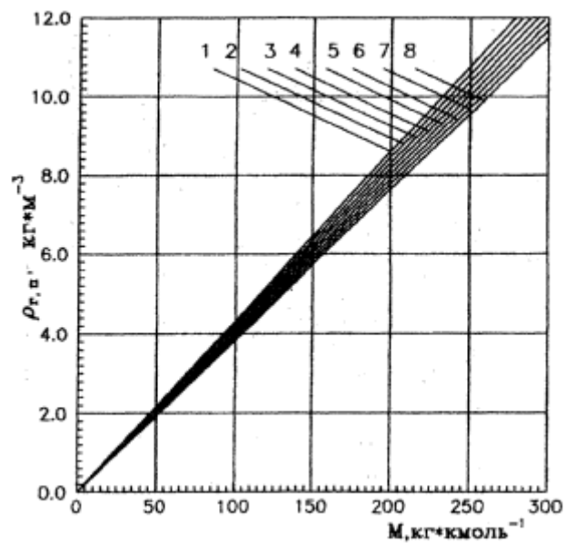
Рис. 3. Зависимость плотности \rho_{г,в} ГГ и паров ПВЖ от молярной массы M при различных расчетных температурах t_p : 1-10 °C; 2-15°C; 3-20 °C; 4-25 °C; 5-30 °C; 6-35 °C; 7-40 °C; 8-45°C
