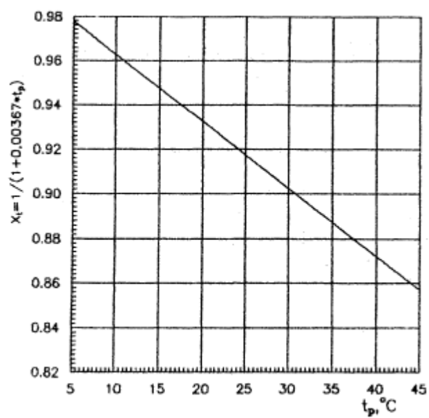
Рис. 2. Зависимость параметра x_t = 1 / (1 + 0,00367 \cdot t_p) от расчетной температуры t_p
