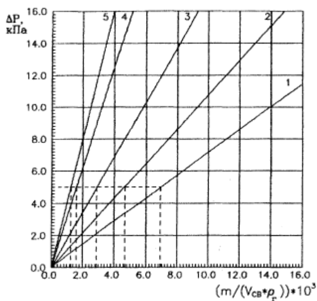
Рис. 17. Зависимость избыточного давления взрыва \Delta P для горючих газов, определенная по формуле (1) НПБ 105-95, от параметра \frac{m}{V_{св} \cdot \rho_r} : 1 - водород ( Z = 1,0 ); 2 - метан ( Z = 0,5 ); 3 - этан ( Z = 0,5 ); 4 - пропан ( Z = 0,5 ); 5 - бутан ( Z = 0,5 )
