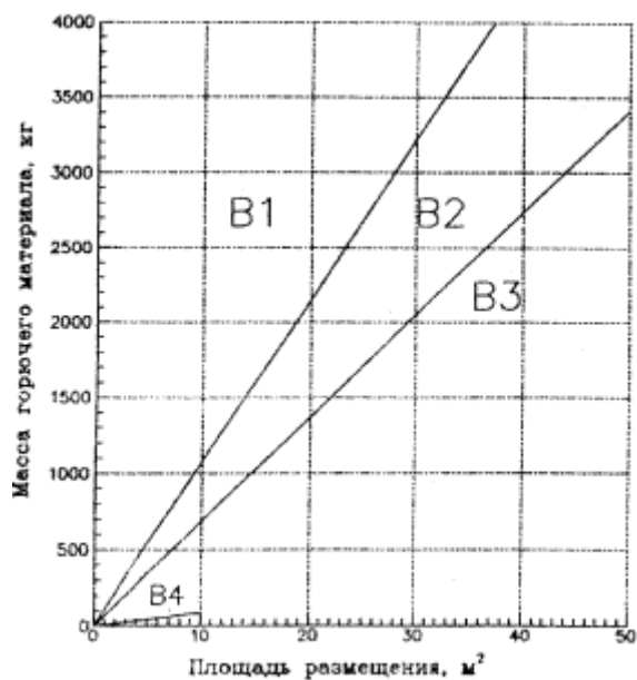
Рис. 39. Определение категорий помещений с шерстью
