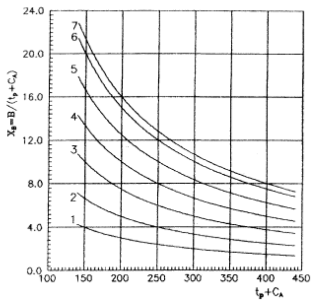
Рис. 7. Зависимость параметра x_s = B/(t_p + C_A) для паров ЛВЖ от параметра (t_p + C_A) при различных значениях параметра B : 1-600; 2-1000; 3-1500; 4-2000; 5-2500; 6-3000; 7-3200
