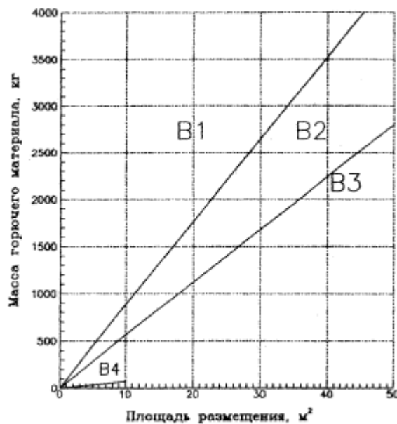
Рис. 33. Определение категорий помещений с бурый углем
