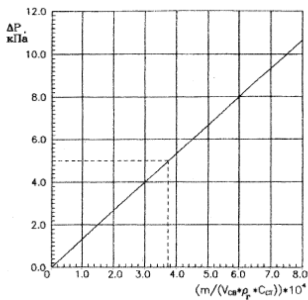
Рис. 16. Зависимость избыточного давления взрыва \Delta P для горючих газов (кроме водорода), определенная по формуле (1) НПБ 105-95, от параметра \frac{m}{V_{св} \cdot \rho_r \cdot C_{ст}} при Z = 0,5
